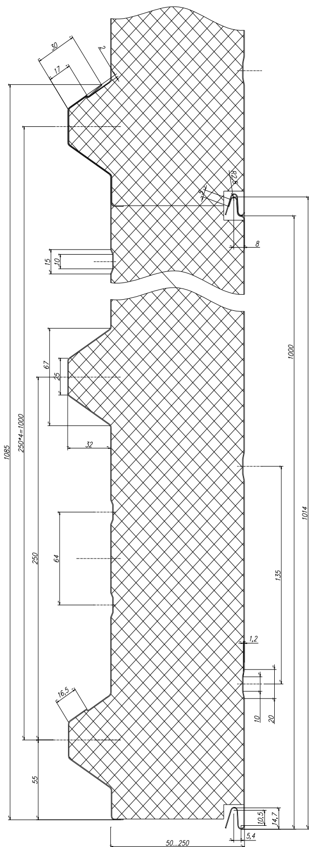
Трехслойная панель кровельная ТПК тип 5
