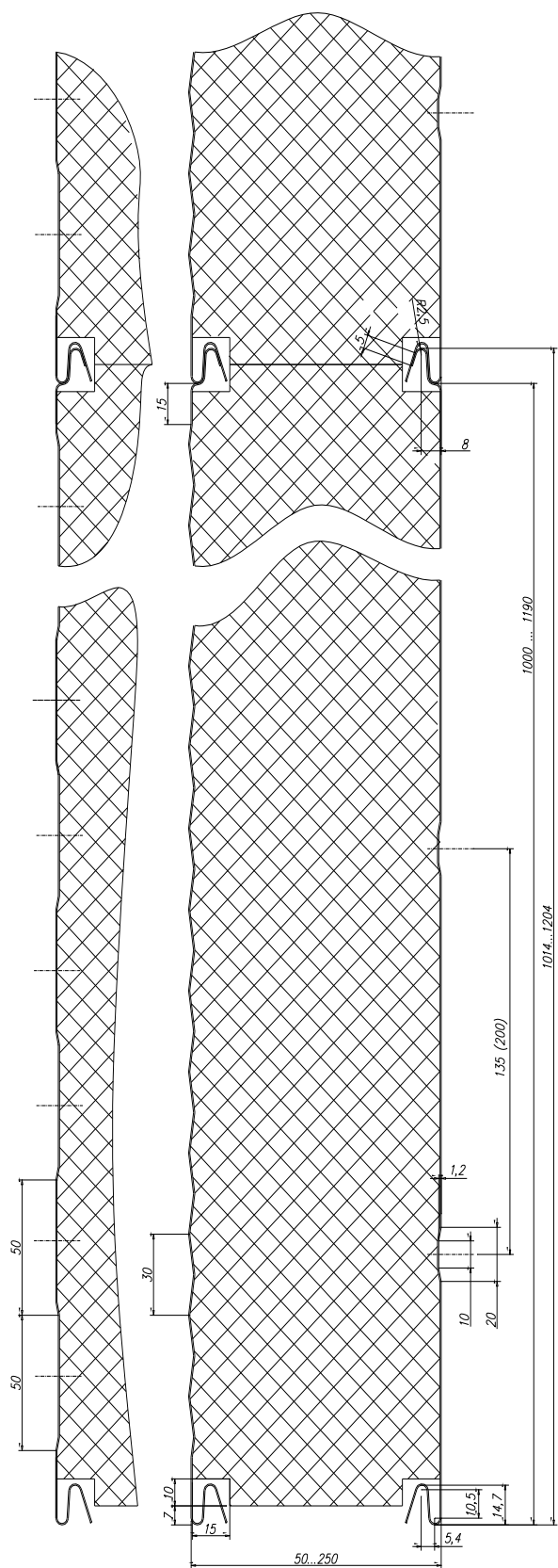
Трехслойная панель стеновая ТПС тип 5
